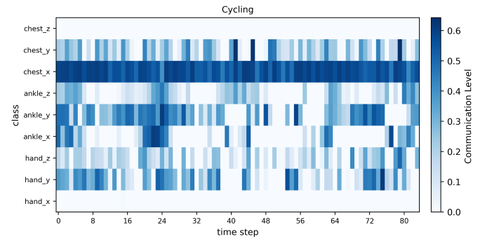
(d) Cycling
