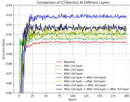
(a) PAMAP2
